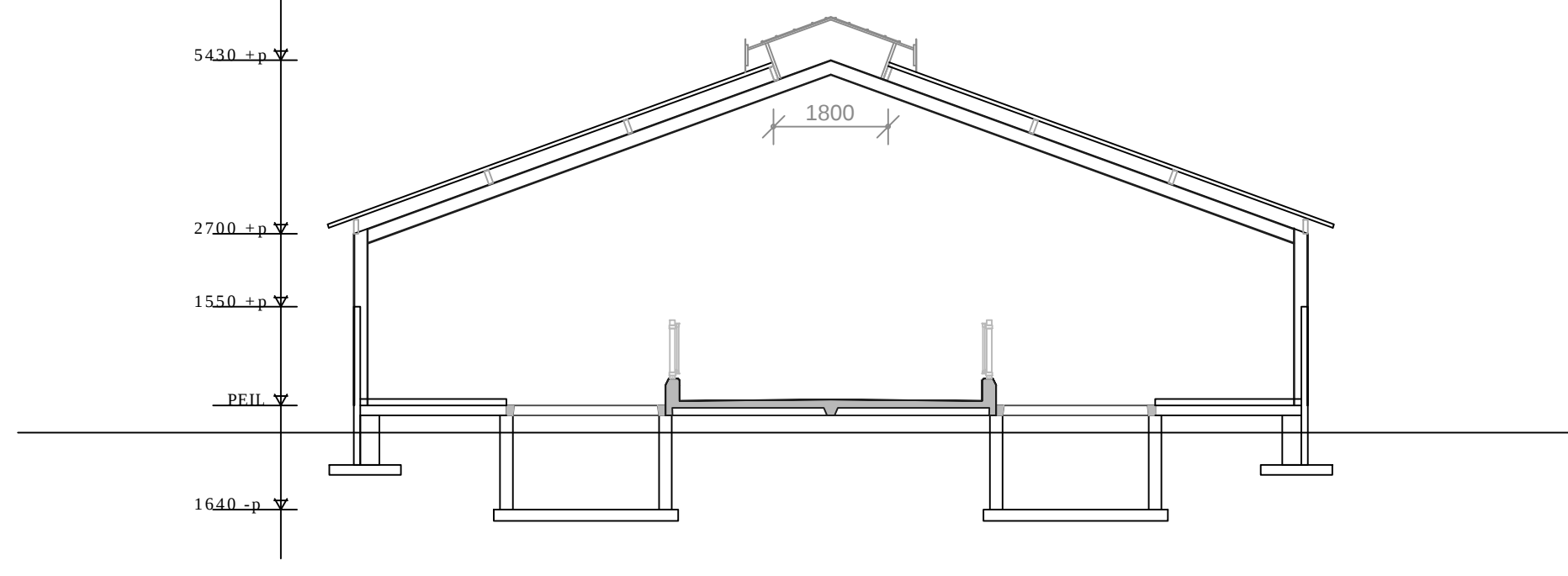
DOORSNEDE B-B
