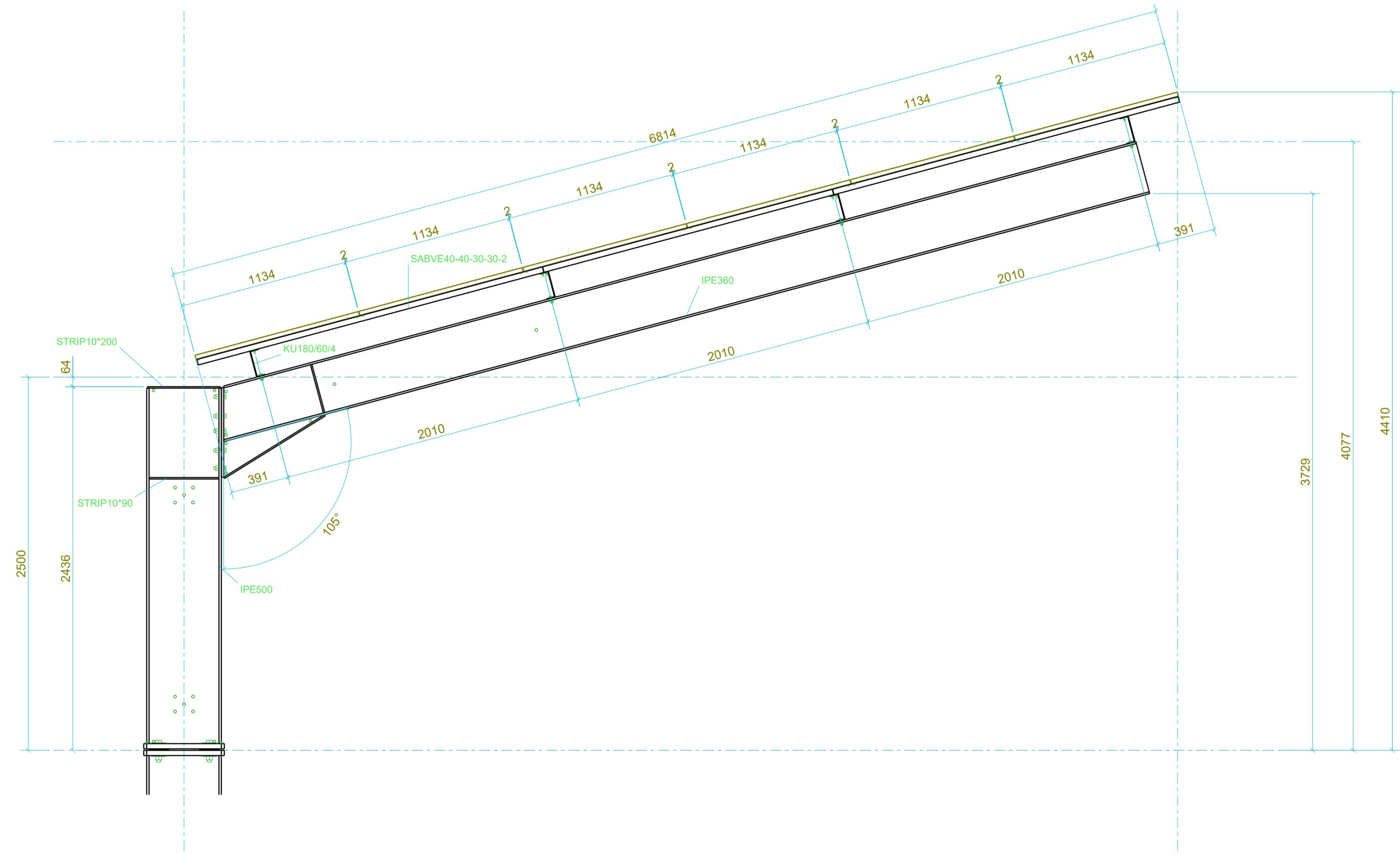
dsn A - A, 1:25
