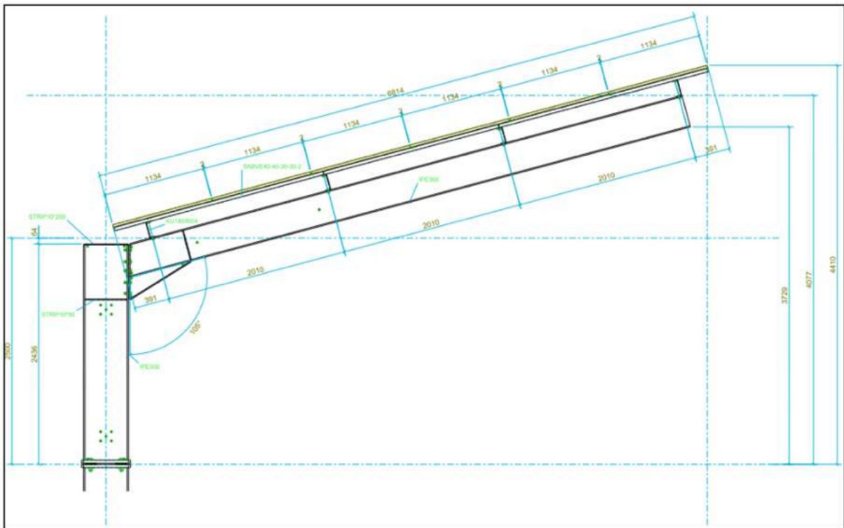
Afbeelding 2.3 Dwarsdoorsnede van de te realiseren carport
