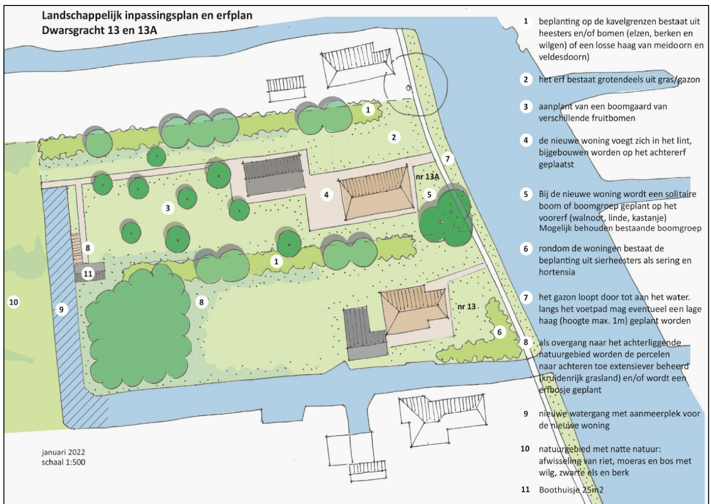
Figuur 1.1 Inpassingsplan met de beoogde watergang (9) en het beoogde woonhuis met boothuis (4 en 11)
