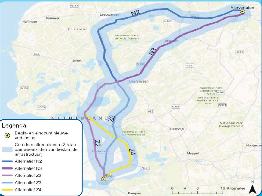
Afbeelding 1: De te onderzoeken tracéalternatieven voor de nieuwe 380 kV-verbinding
