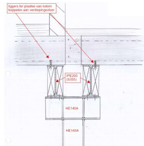
figuur 2. Wijziging draagconstructie
