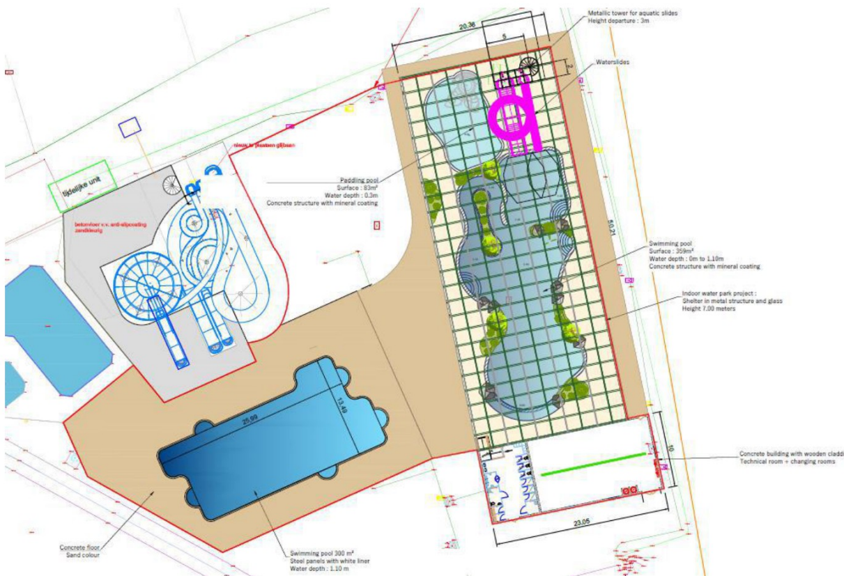
Figuur 2 – Inrichting planlocatie.
