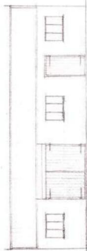
R. Zijgevel.
