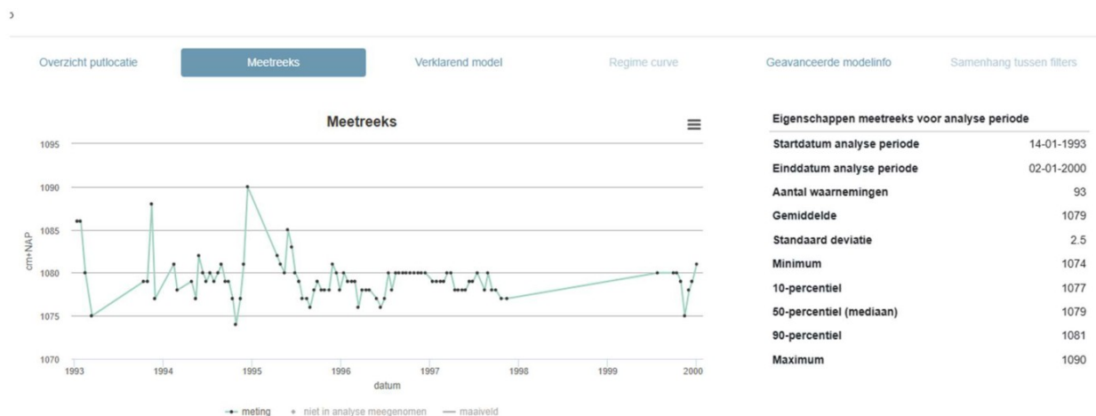
Figuur 2: Verloop grondwaterstand
