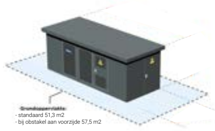
DR (station maat: 6,4 x 2,5 x 2,41m, kavelmaat: 10,32 x 4,97m)
