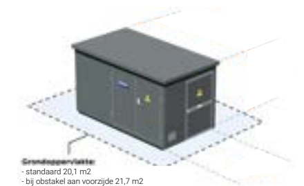
Alfen Pacto 25 (station maat: 3,55 x 1,76 x 2,06m, kavelmaat: 5,22 x 3,85m)
