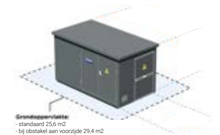
Alfen Pacto 30 (station maat: 3,65 x 1,99 x 2,06m, kavelmaat: 6,42 x 3,99m)
